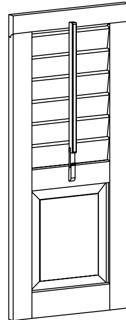
Ladentyp: Füllungsladen einseitig abgeplattete Füllung 18mm und bewegliche Lamellen 100 mm
