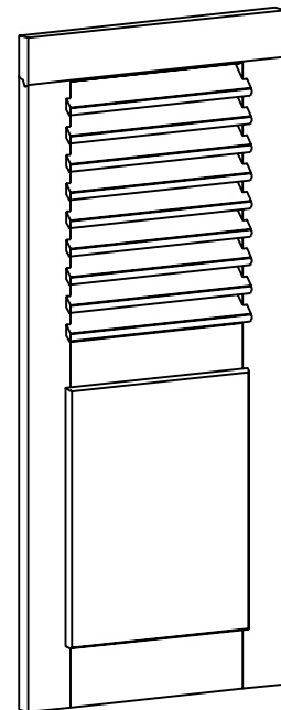
Ladentyp: Füllungsladen überschobene Füllung 33 mm und feste Rhomboidlamelle 70Rp
